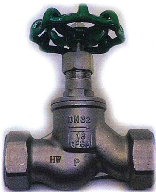
HW.J11W-16RDN15 / HW.J11W-16RDN20 / HW.J11W-16RDN25 / HW.J11W-16RDN32 / HW.J11W-16RDN40 / HW.J11W-16RDN50
